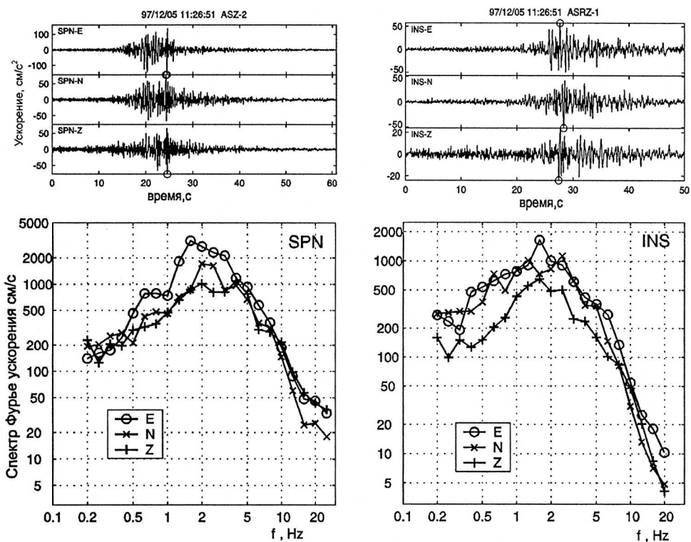
Рис. 11. Акселерограммы Кроноцкого землетрясения по записям сейсмических станций "Шипунский" и "Институт" и ниже их сглаженные спектры Фурье
