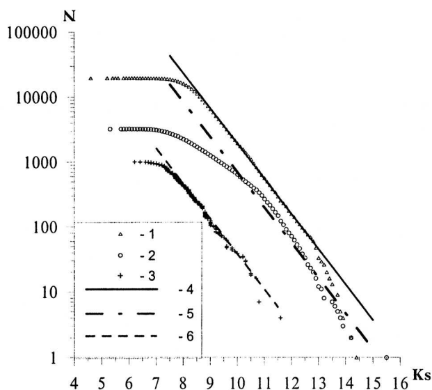
Рис. 2. Кумулятивные графики повторяемости землетрясений в районе Кроноцкого очага
