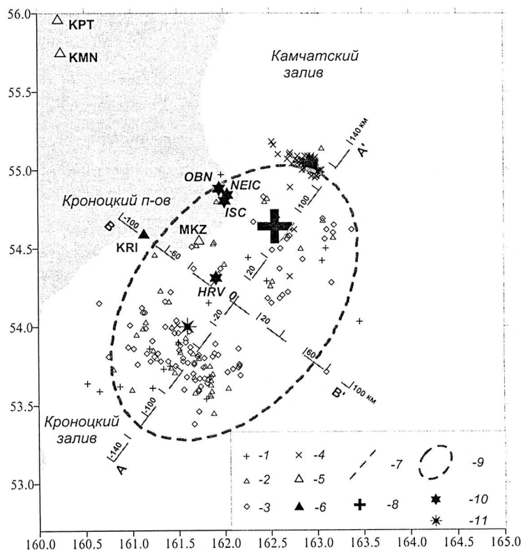
Рис. 4. Карта эпицентров афтершоков Кроноцкого землетрясения, происшедших 5 декабря (в первые восемь часов)
