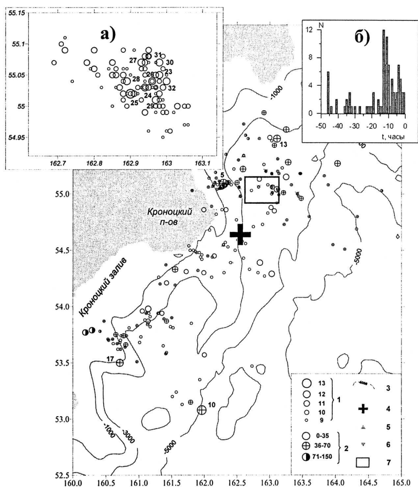
Рис. 3. Карта эпицентров землетрясений за 01.12.-02.12.1997 г.
