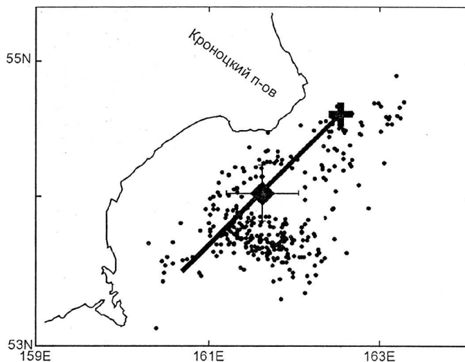
Рис. 7. Результаты восстановления пространственных характеристик высокочастотного (0.5-2.0 Гц) очага Кроноцкого землетрясения по телесеismicическим записям Р-волн
