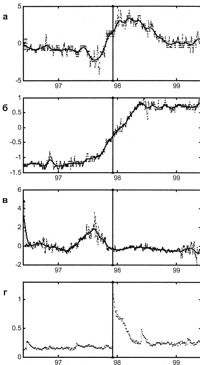
Рис. 16. Примеры аномальных вариаций режима подземных вод в связи с Кроноцким землетрясением
