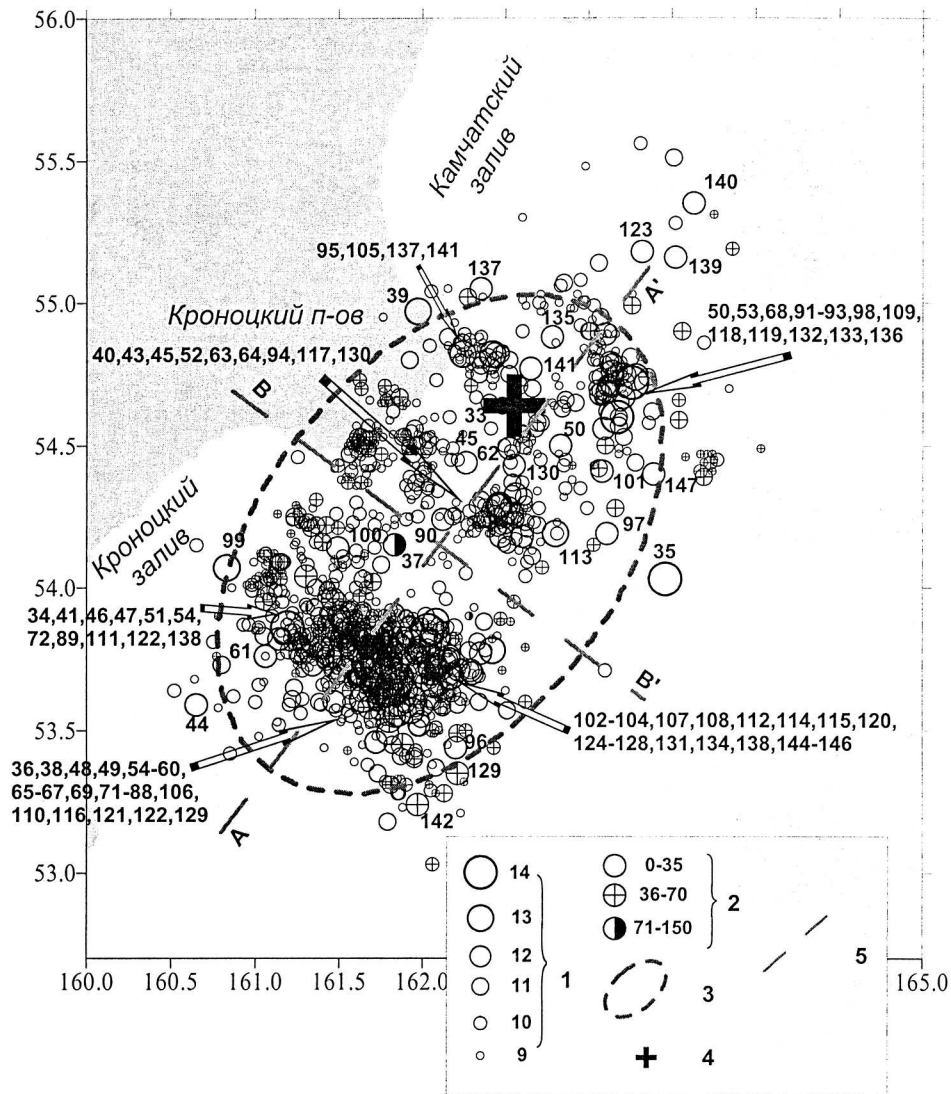
Рис. 5. Карта эпицентров всех афтершоков Кроноцкого землетрясения
