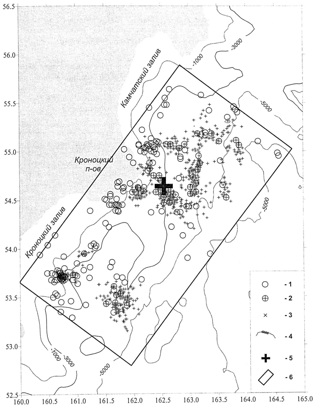
Рис. 1. Карта эпицентров землетрясений района очага Кроноцкого землетрясения за 1962-1996 гг.
