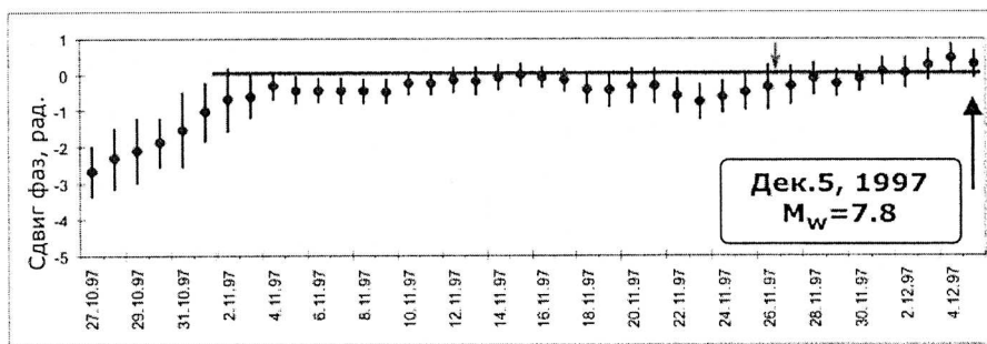
Рис. 17. Вариации фазы компоненты ВСШ, соответствующей приливной волне O_1 перед Кроноцким землетрясением
