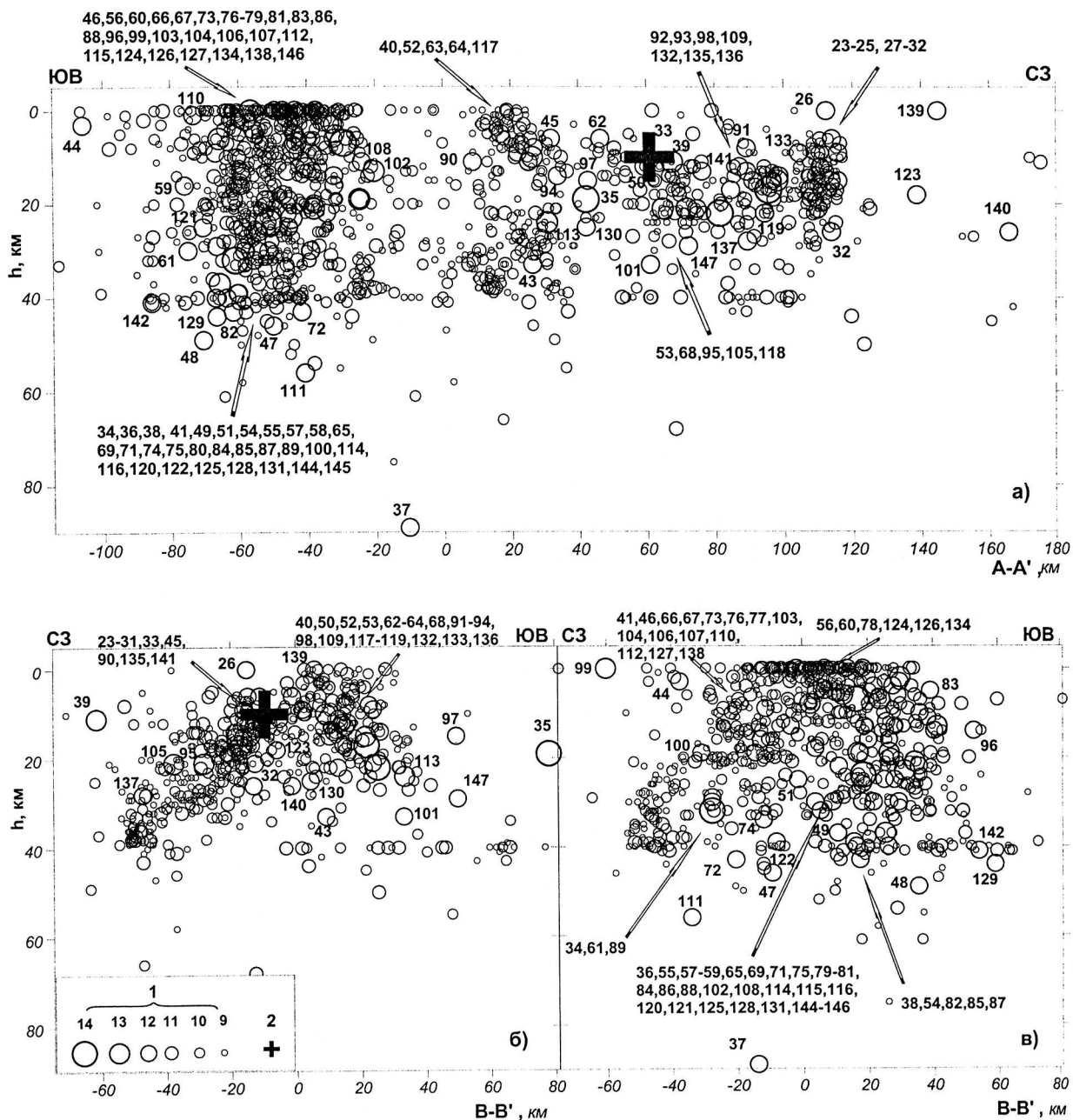
Рис. 6. Вертикальные разрезы совокупности афтершоков Кроноцкого землетрясения
