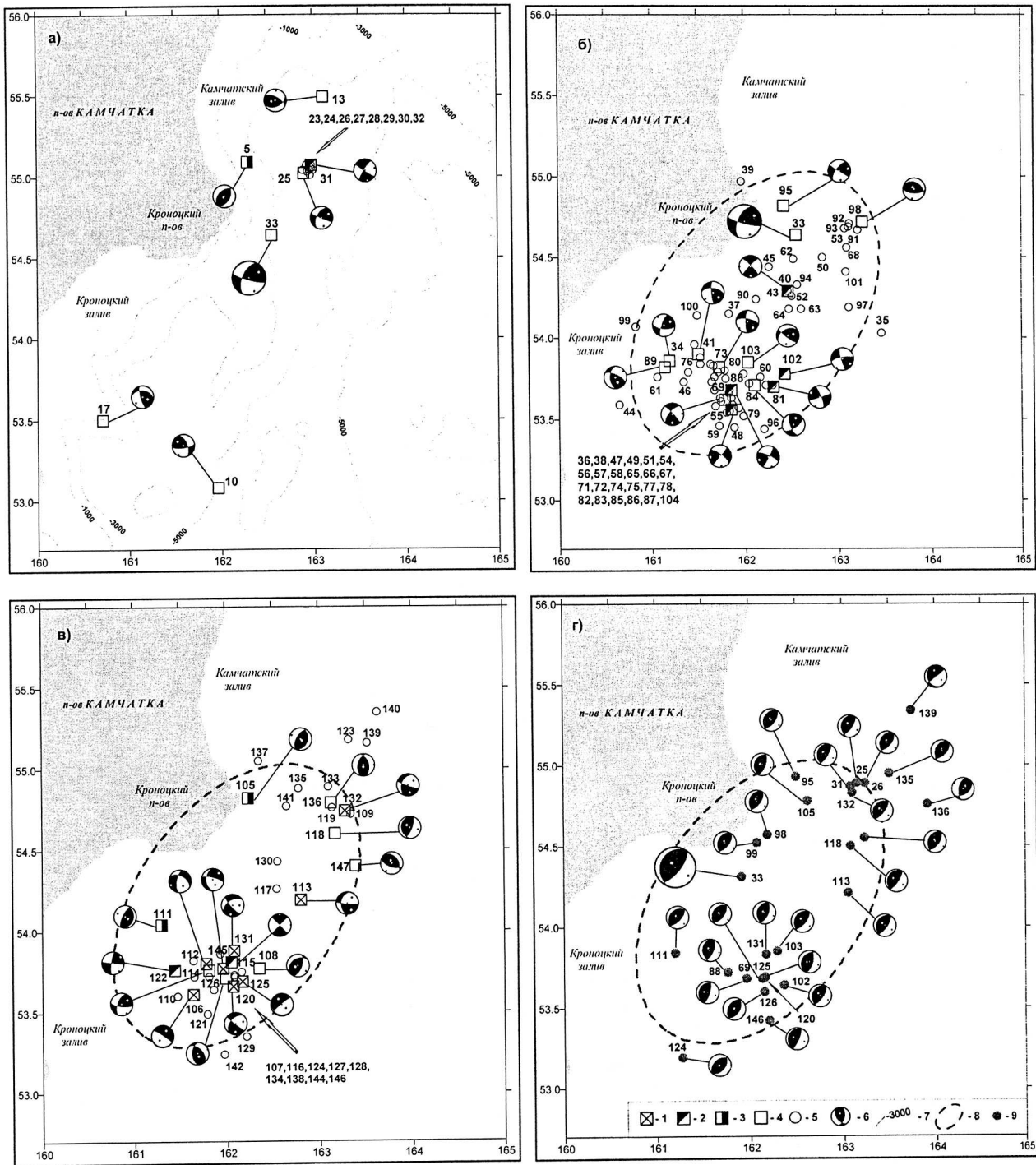
Рис. 8. Карта механизмов очагов сильных ( K_S \geq 11.6 ) землетрясений района очага Кроноцкого землетрясения за разные периоды времени: с 01.01.1997 г. по 11 h 27 m 5 декабря (а); за первые сутки после основного толчка (б); 06.12.-31.12.1997 г. (в); по каталогу [5] за 05.12.-31.12.1997 г. (г).
