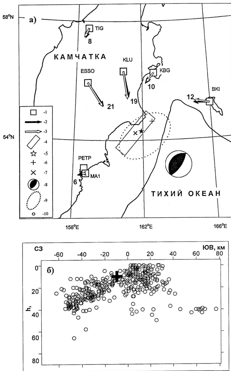
Рис. 14. Результаты восстановления характеристик статического очага Кроноцкого землетрясения по косейсмическим смещениям (горизонтальные компоненты), зарегистрированным GPS-станциями: положение статического очага и вектора горизонтальных смещений относительно станции "Петропавловск Камчатский" (а); проекции на вертикальную плоскость, ориентированную вкост фокальной зоны, гипоцентров афтершоков за период 5-31 декабря, в определении координат которых обязательно участвовали фазы Р- и S-волн на ближайшей к очагу станции (б).
