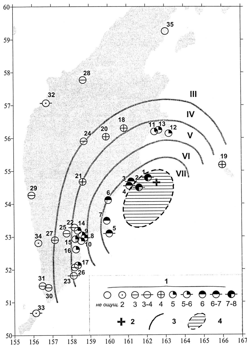
Рис. 9. Карта изосейст Кроноцкого землетрясения 05.12.1997 г. в 11 h 26 m с M_w=7.8
