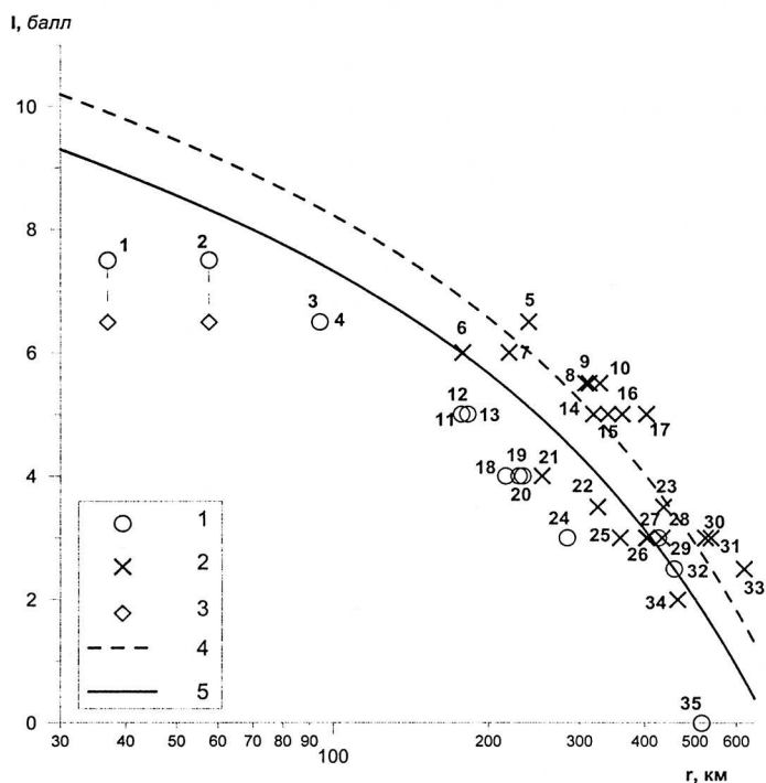
Рис. 10. График затухания интенсивности сотрясений
