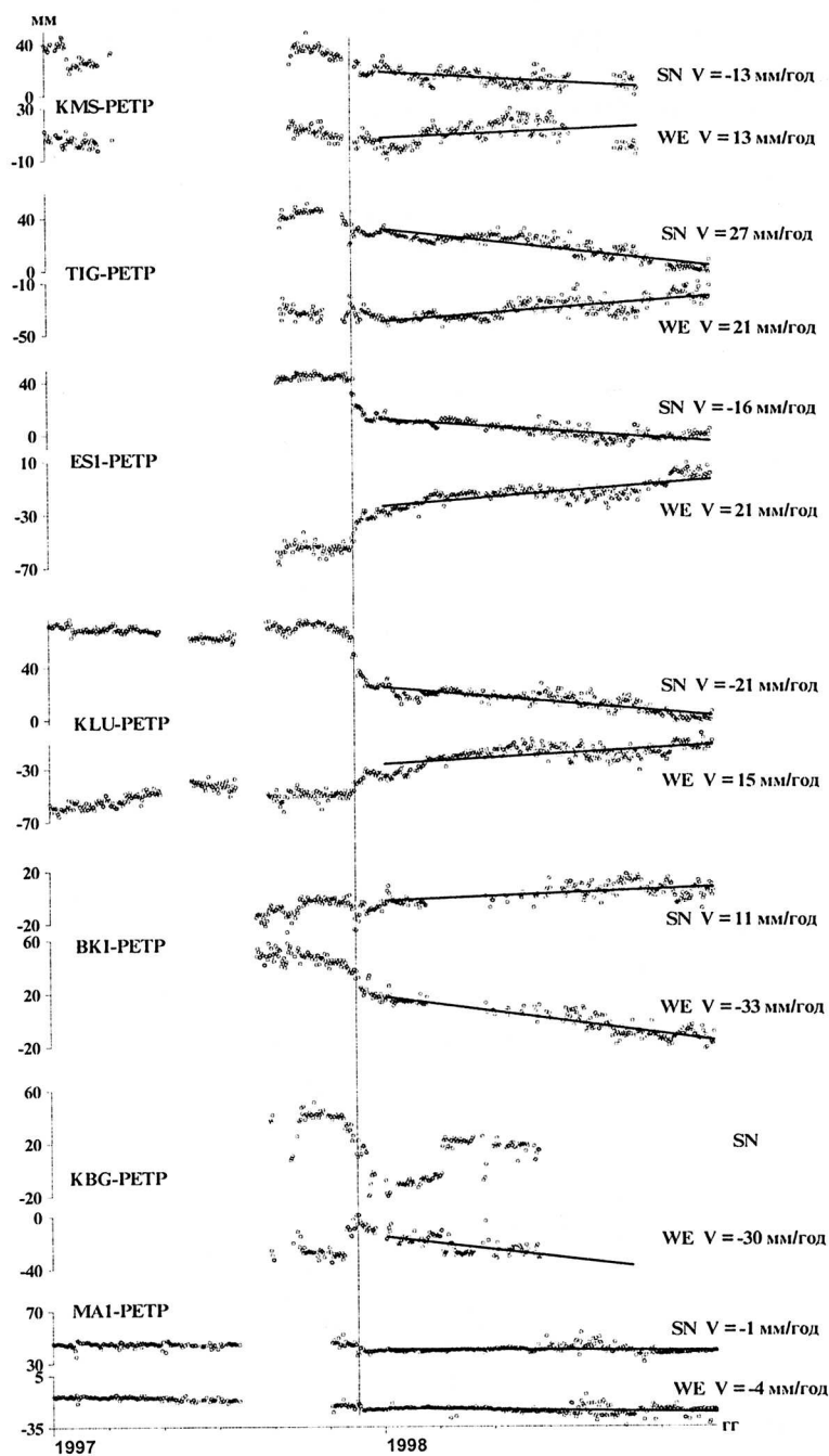
Рис. 13. Смещения пунктов относительно станции "Петропавловск-Камчатский" по направлениям север-юг (NS) и запад-восток (WE)
