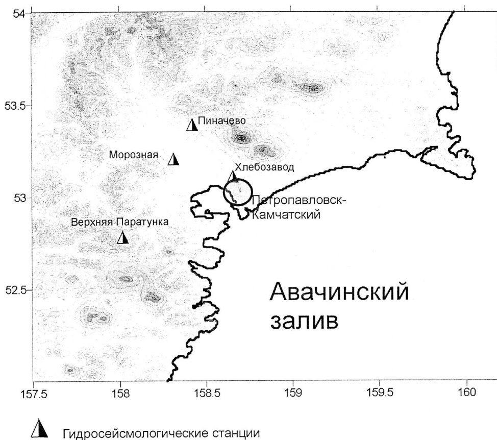
Рис. 15. Схема сети гидрогеологических станций Камчатского полигона
